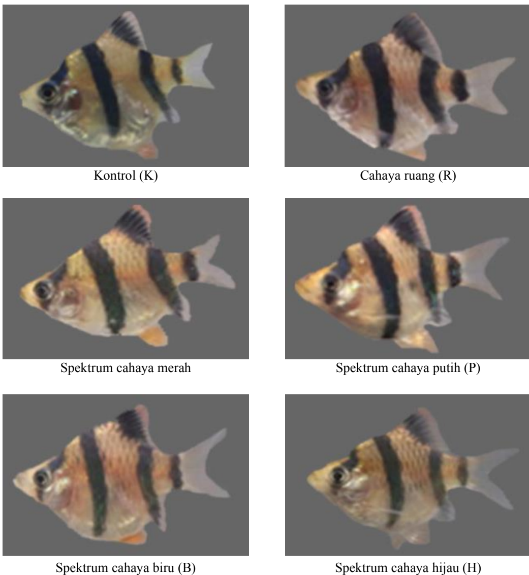
Gambar 2 Pengamatan kualitas warna ikan sumatra Puntigrus tetrazona dengan perlakuan paparan spektrum cahaya berbeda menggunakan kamera DSLR.
